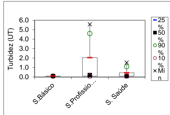
Gráfico 13. Turbidez nas amostras dos bebedouros da UFPA
