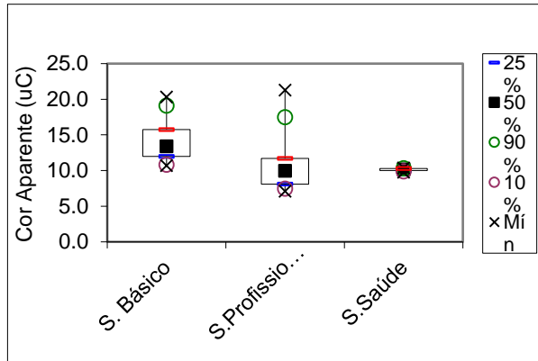
Gráfico 12. Cor aparente das amostras dos bebedouros da UFPA
